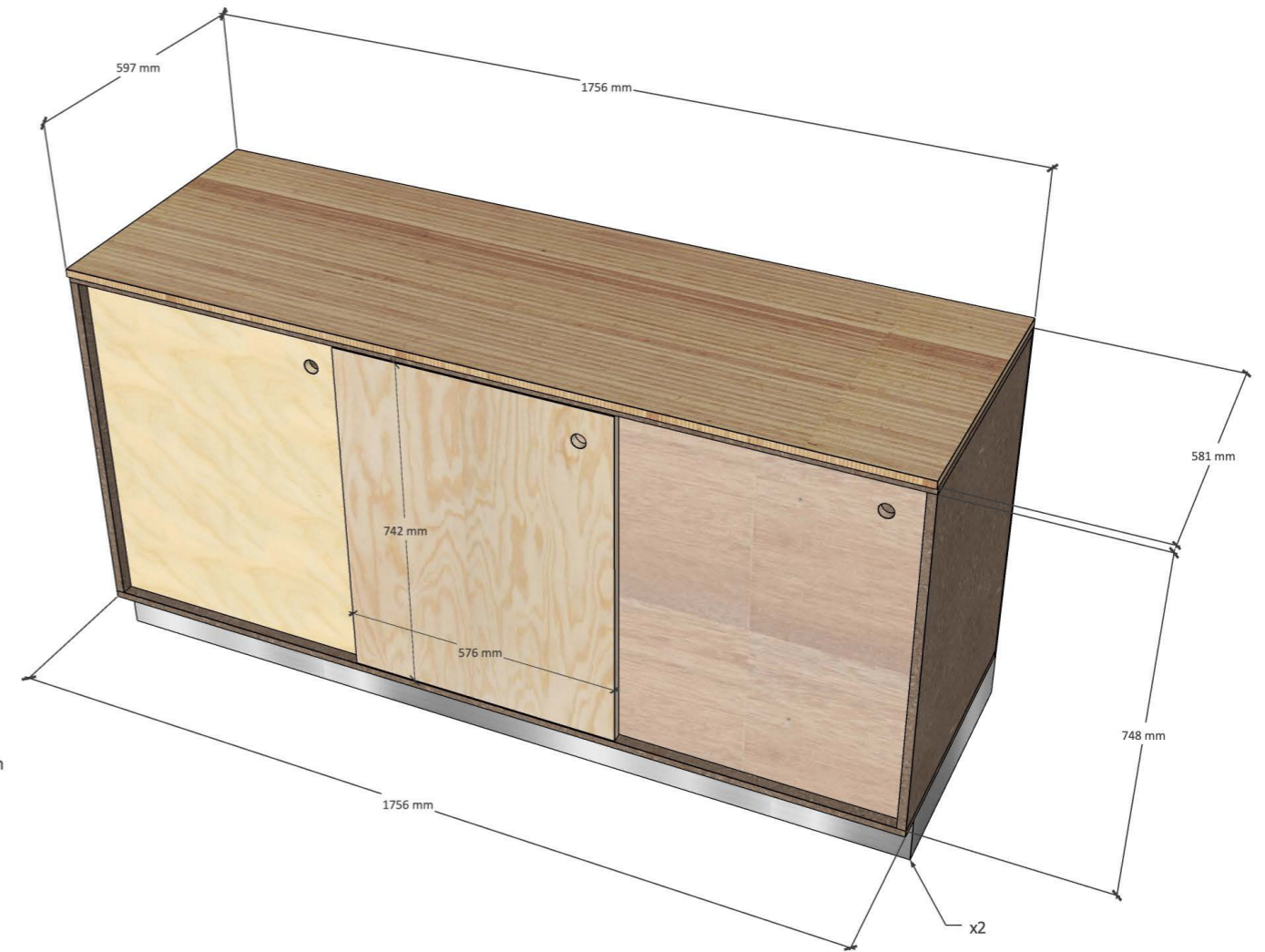
DB_met fronten
