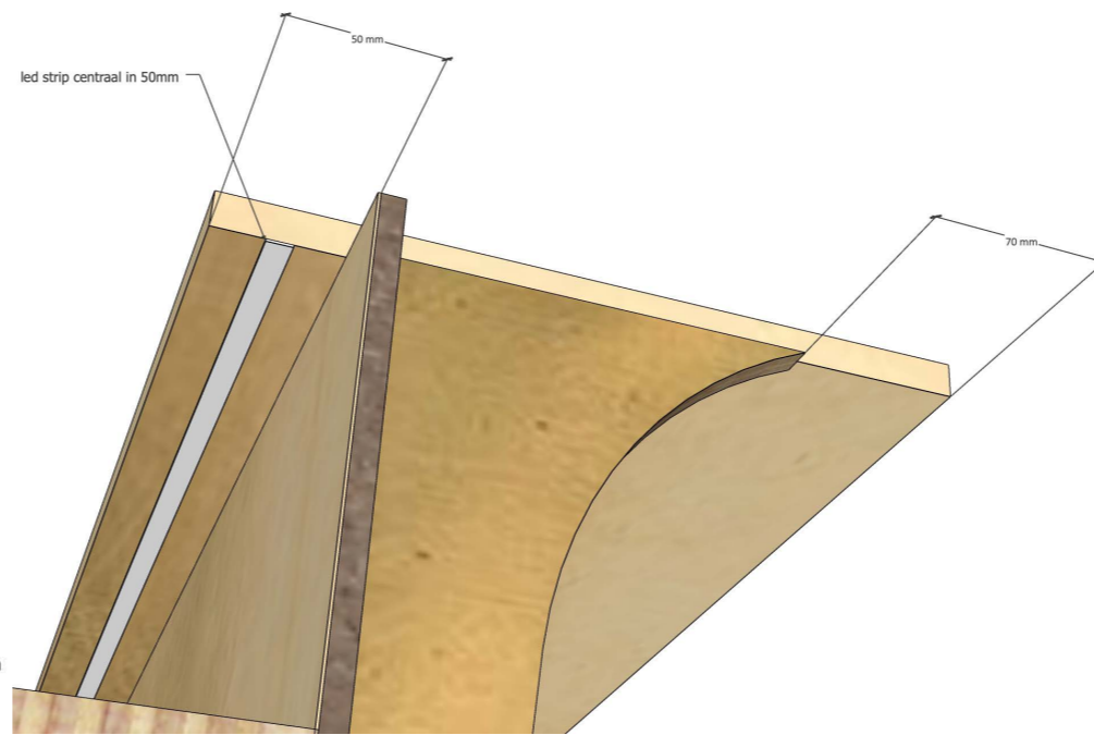
DE_detail hoe toog aansluit op rug en tevens spatwand (CM platen komen ertussen te liggen)
