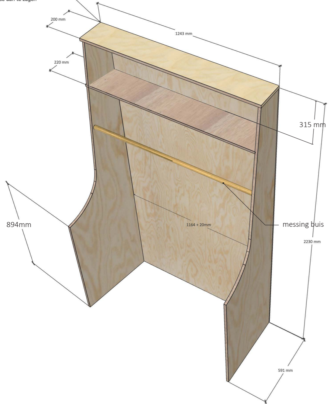
DA_overzicht
