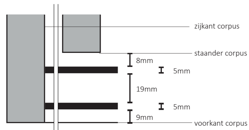
Details infrezing voor schuifdeuren
